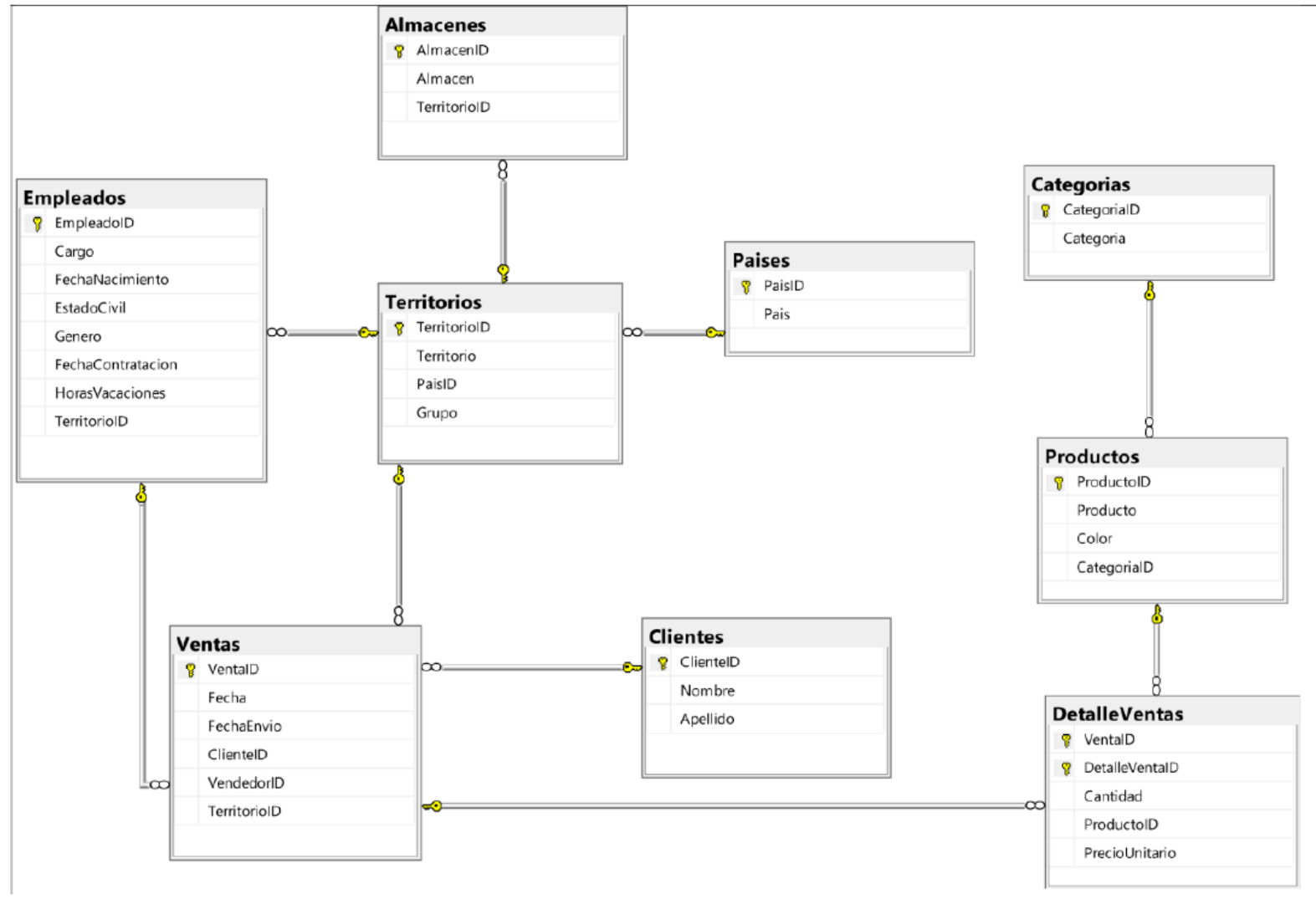
(Figura1): Modelo Relacional BikeZ.
